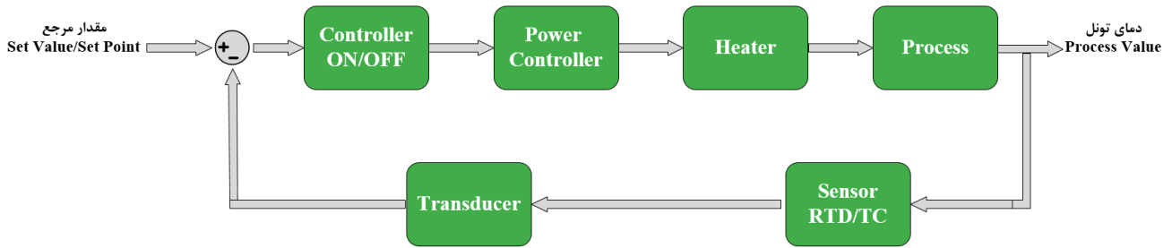
شکل ۳-۴ بلوک دیاگرام کنترل دو وضعیتی
