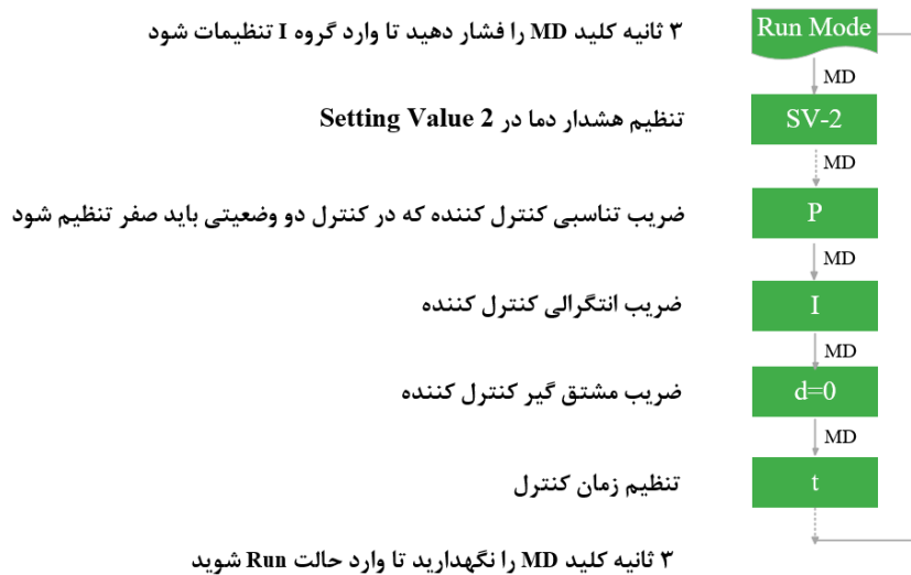
شکل ۱-۵ تنظیم کنترل کننده برای کنترل تناسبی - انتگرالی
