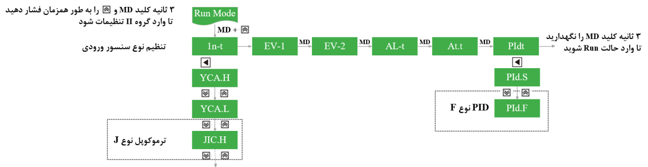
شکل ۴-۳ تنظیم نوع کنترل کننده PID در تجهیز Autonics
