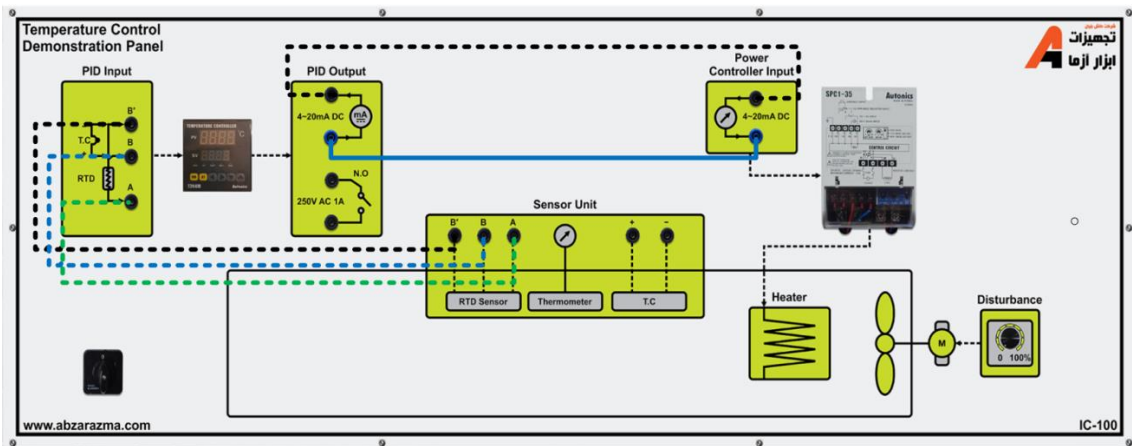
شکل ۳-۶ نحوه سیم‌بندی آزمایش کنترل دو وضعیتی
