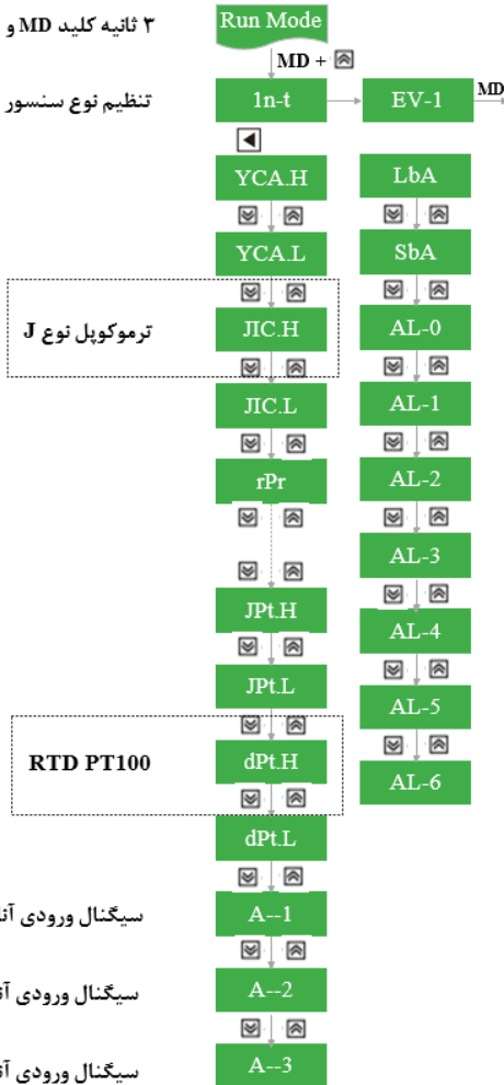
شکل ۳-۵ نحوه انتخاب نوع سنسور
