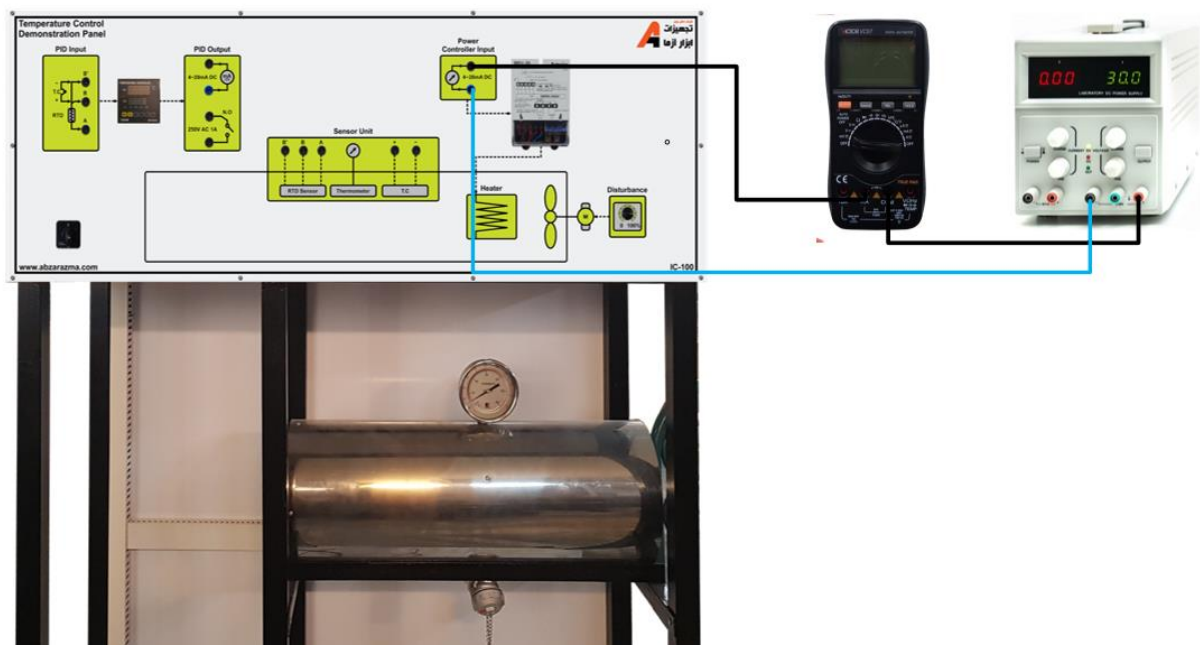
شکل ۲-۱ نحوه پیاده‌سازی آزمایش کنترل حلقه باز فرآیند تونل هوای گرم
