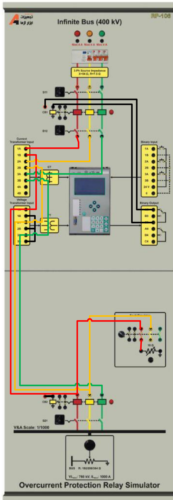
شکل ۱-۲ نحوه پیاده‌سازی آزمایش حفاظت اضافه جریان با رله وبکو
